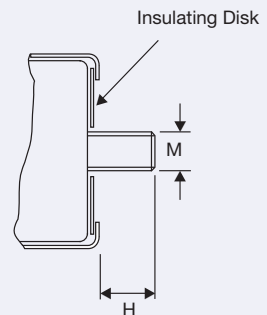
ALS37 Stud Mounting
